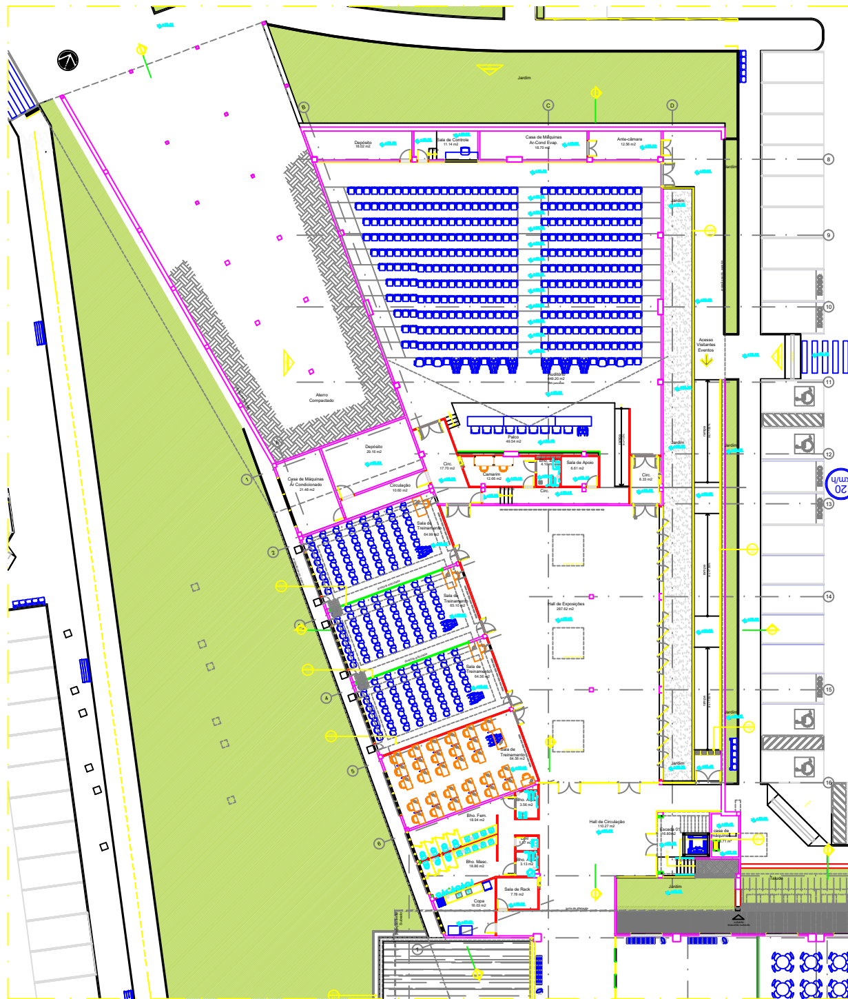
01 Planta de Layout - Térreo Eventos
